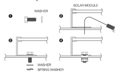
Рисунок 1. Монтаж болтами
